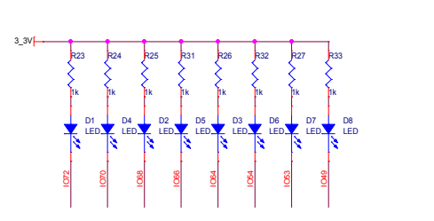
发光二极管模块
