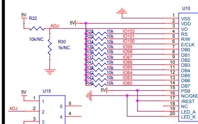
12864/1602 液晶接 口
