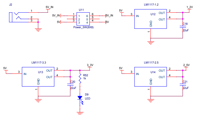
LDO 电 源
