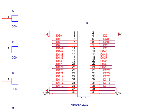
扩展接 口（兼容黑金开发 板）
