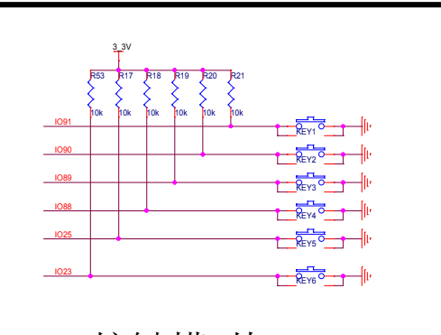
按键模 块
