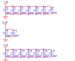
电源滤波退耦电 路
